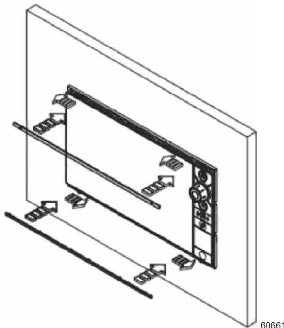
Montering av infattning, avlägsna genom att göra tvärtom
